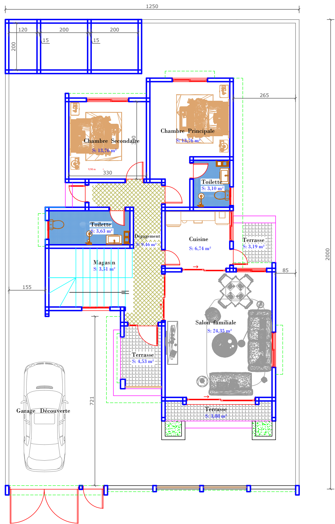
SURFACE TOTALE: 91 m² PLAN DU REZ DE CHAUSSEE
